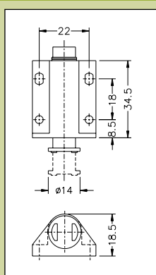
Magnet na pritisak - jednodelni
