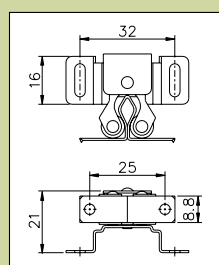
Prava ringlica sa prihvatnikom
