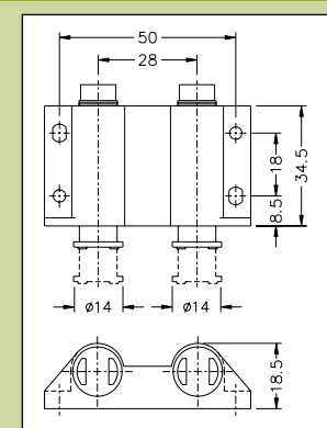
Magnet na pritisak - dupli
